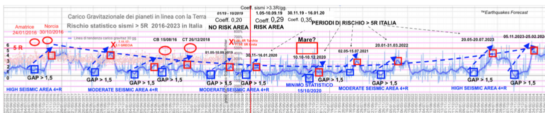
Grafico A della probabilità statistica da motivazioni astronomiche, per terremoti >5R in ITALIA nel periodo 2016-2023
